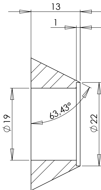
SECTION A-A
